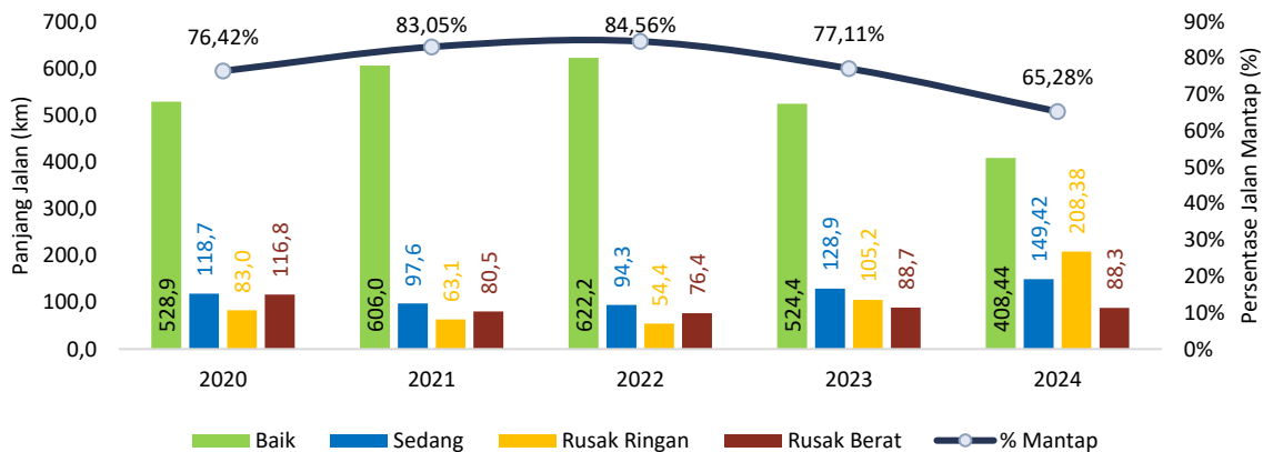
Gambar 2. 44 Grafik Kondisi Jalan Kabupaten Tegal Tahun 2020-2024
