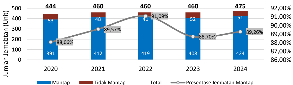
Gambar 2. 46 Grafik Kondisi Jembatan Kabupaten Tegal Tahun 2020-2024
