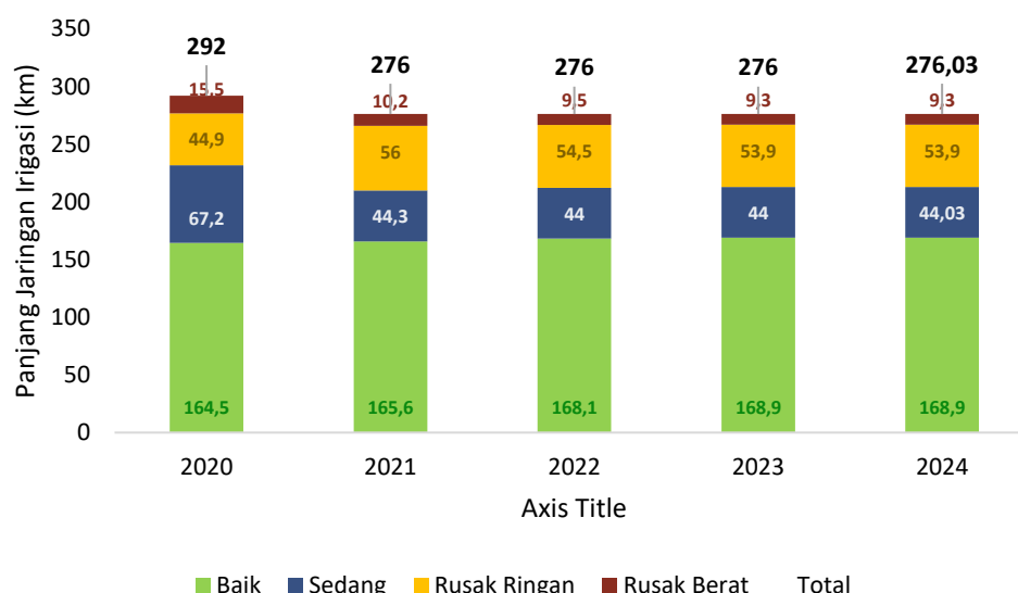
Gambar 2. 39 Grafik Kondisi dan Panjang Jaringan Irigasi Kabupaten Tegal Tahun 2020-2024 2) Infrastruktur Air Minum
