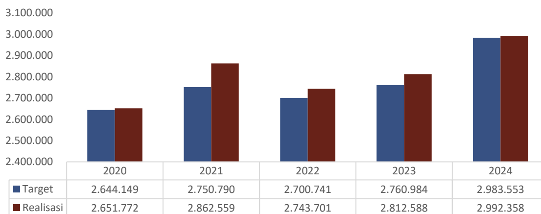
Gambar 2. 46 Target dan Realisasi Pendapatan Daerah Tahun 2020-2024
